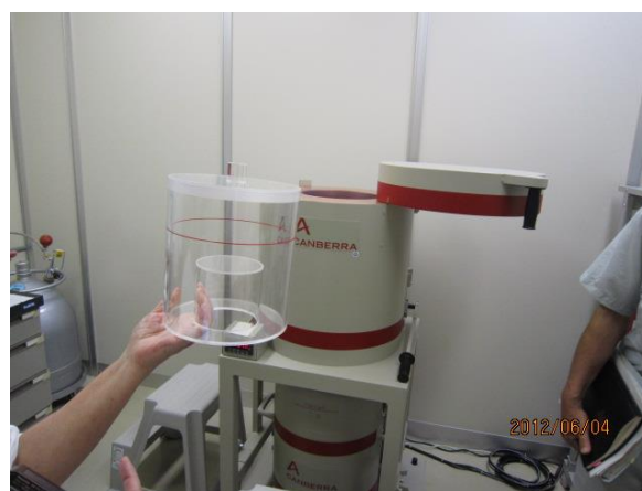
君津広域水道企業団に設置されている測定器 水、水を浄化する途中でできた汚泥の放射線 量を定期的に検査。この容器で水を検査。木更 津市の浄水場6カ所、配水場1カ所の水も毎月 ここで測定。
